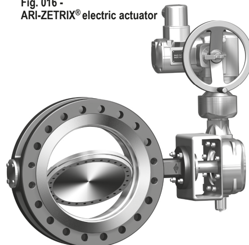
Fig. 016 - ARI-ZETRIX® electric actuator
